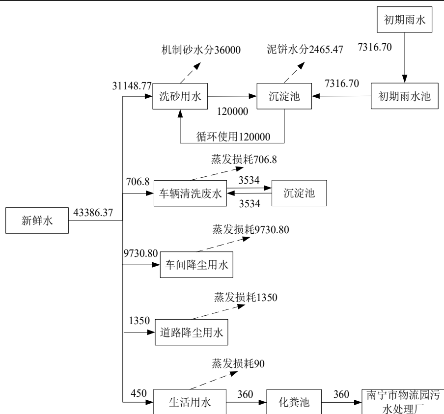
图 2-1 项目运营期水平衡图，单位 \text{m}^3/\text{a}
