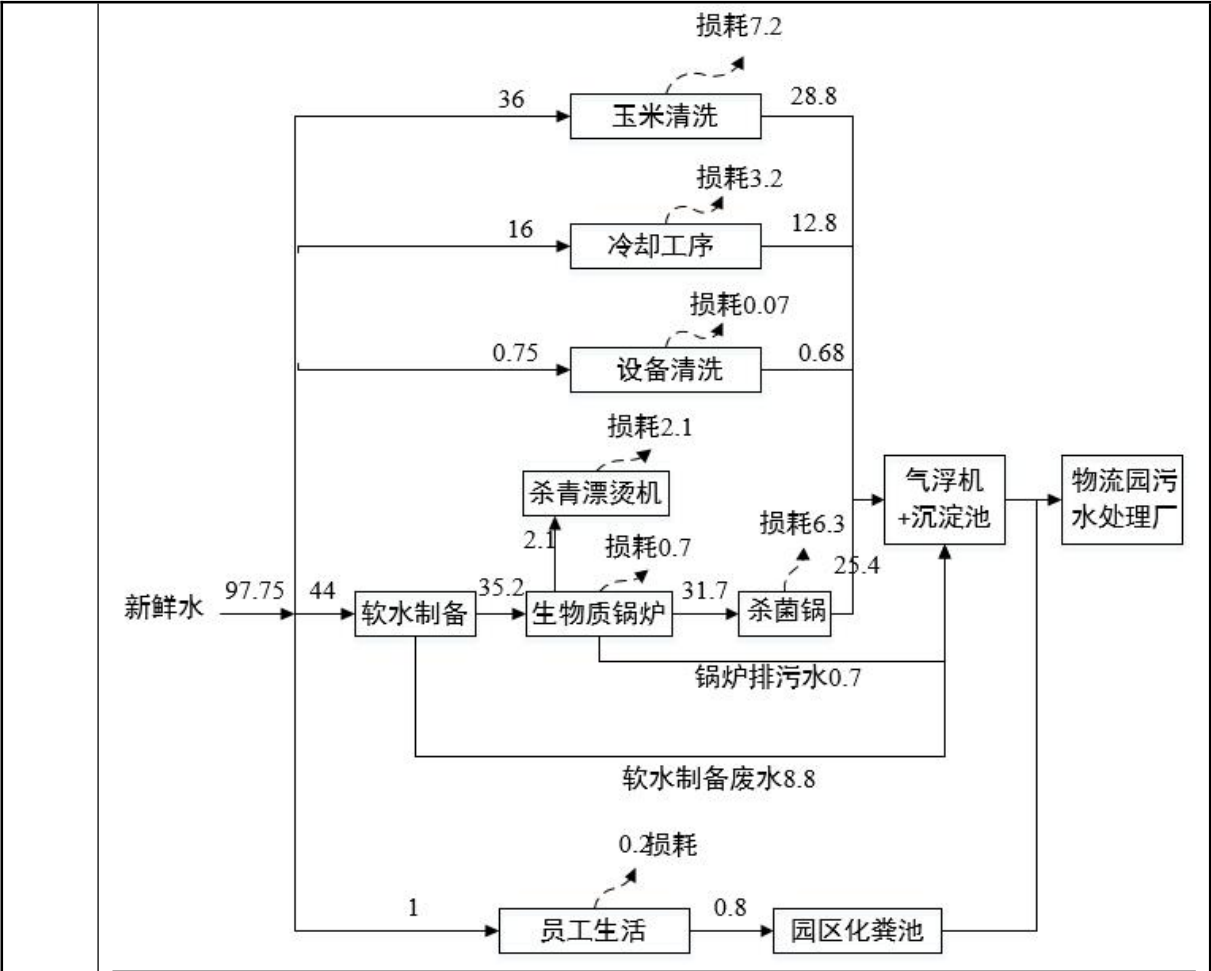
图 2-1 项目水平衡图 单位: \text{m}^3/\text{d}
