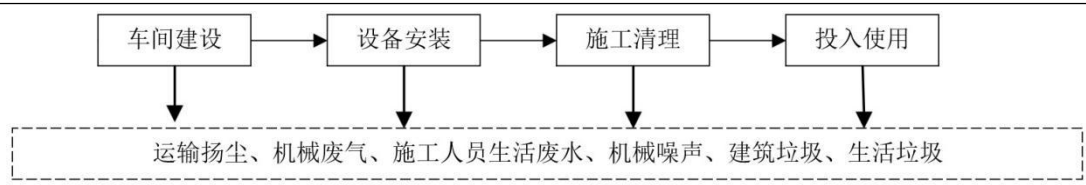
图 2-2 施工期工艺流程图及产污节点图
