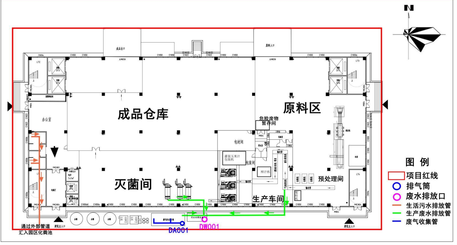
附图2 项目总平面布置图
