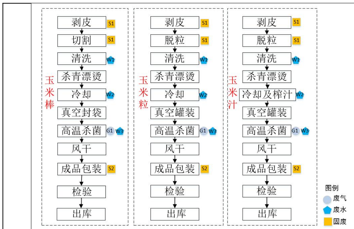
图 2-3 营运期工艺流程图及产污节点图
