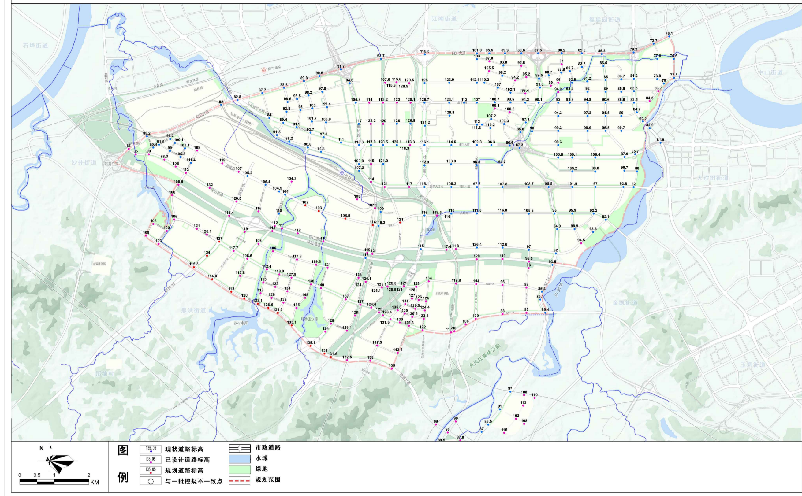
S-19道路竖向规划总图
